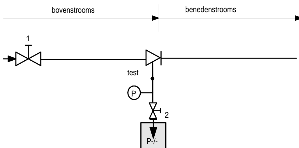
Figuur 2 Controleopstelling vacuümmethode
